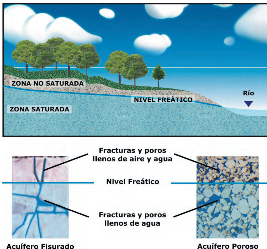
Fig. 4. Zona saturada y no saturada
