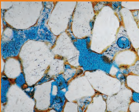
Fig. 11. Microfotografía de arenisca de la Formación Rivera. Clastos de cuarzo con pátina de hematita sobre la superficie. Los poros se encuentran ocupados por resina azul
