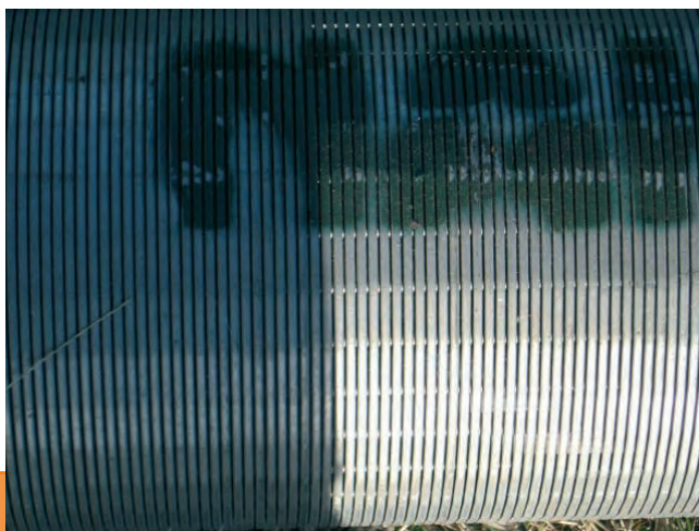
Fig. 25. Filtro de ranura continua. En acero inoxidable, galvanizado o acero crudo. Largo hasta 6 m.
