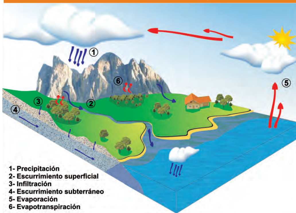
Fig. 1. Componentes del ciclo hidrológico
